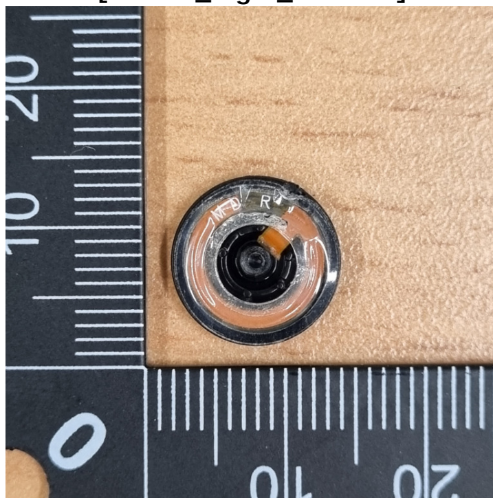
[Earbud_Right_Antenna]
