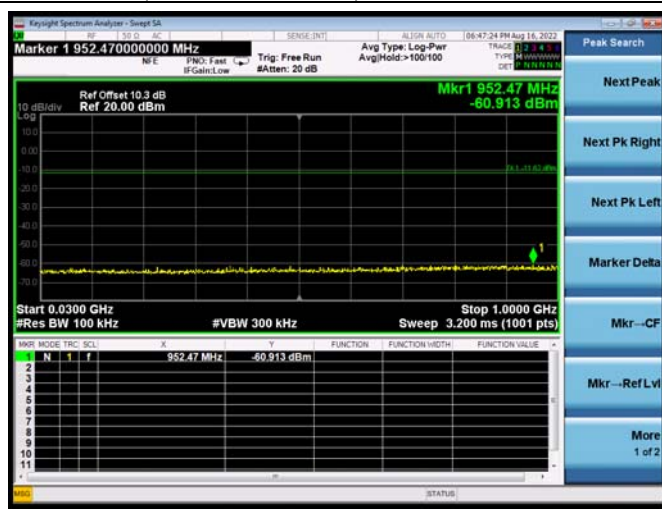
2440MHz(30MHz – 1GHz)
