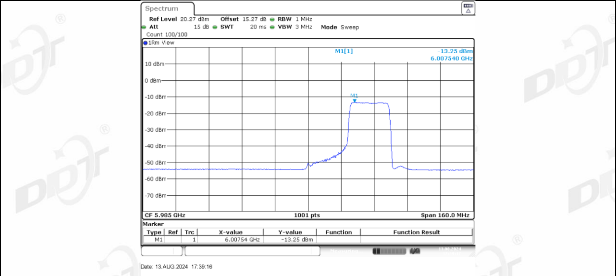
11AX80MIMO_Ant-3_5985_484Tone_RU65
