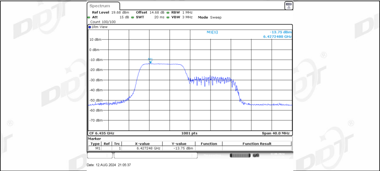
11AX20MIMO Ant-3 6435 106Tone RU54
