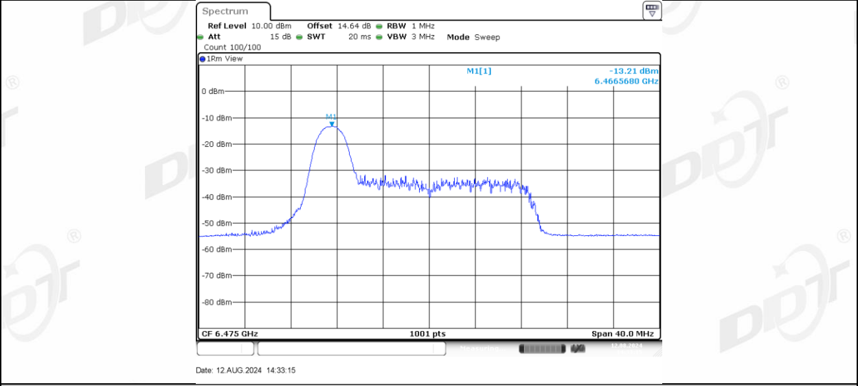
11AX20MIMO Ant-1 6475 26Tone RU4
