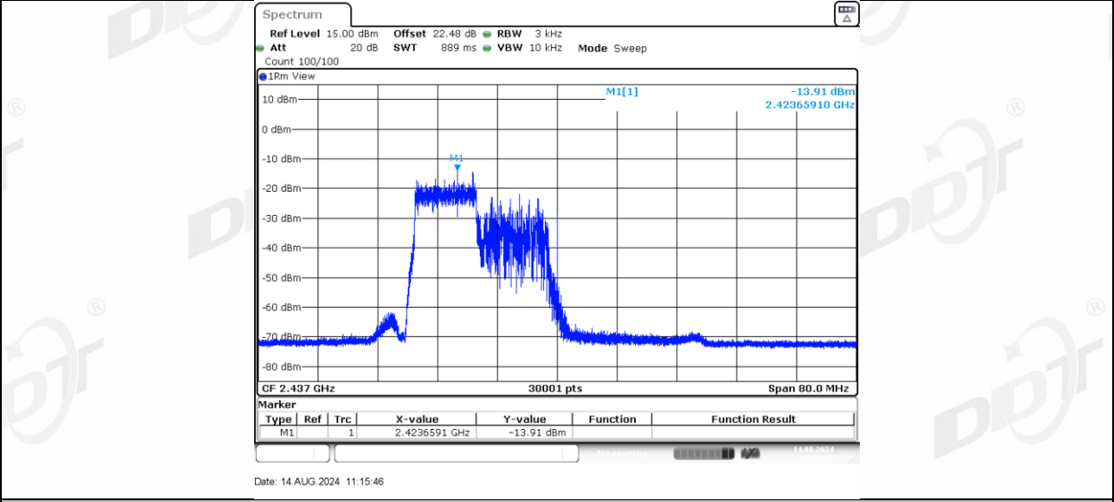
11AX40MIMO_Ant-1_2437_106Tone_RU56
