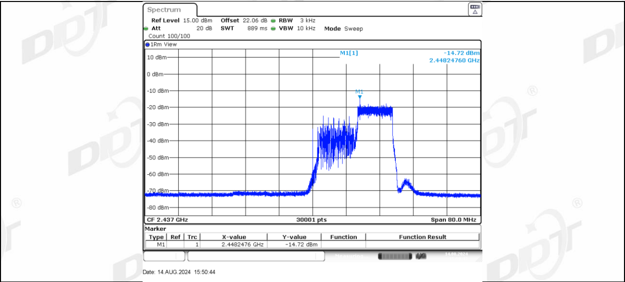
11AX40MIMO_Ant-1_2437_242Tone_RU61
