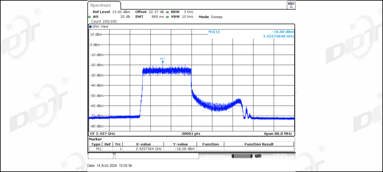
11AX40MIMO_Ant-1_2437_242Tone_RU62
