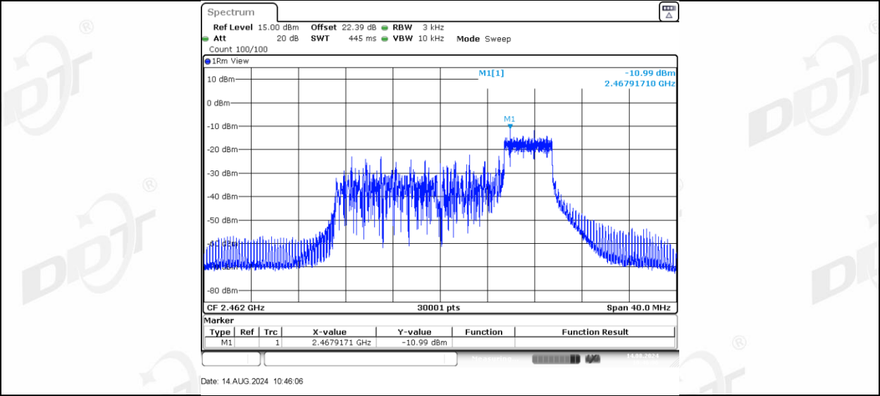
11AX20MIMO_Ant-1_2462_106Tone_RU53
