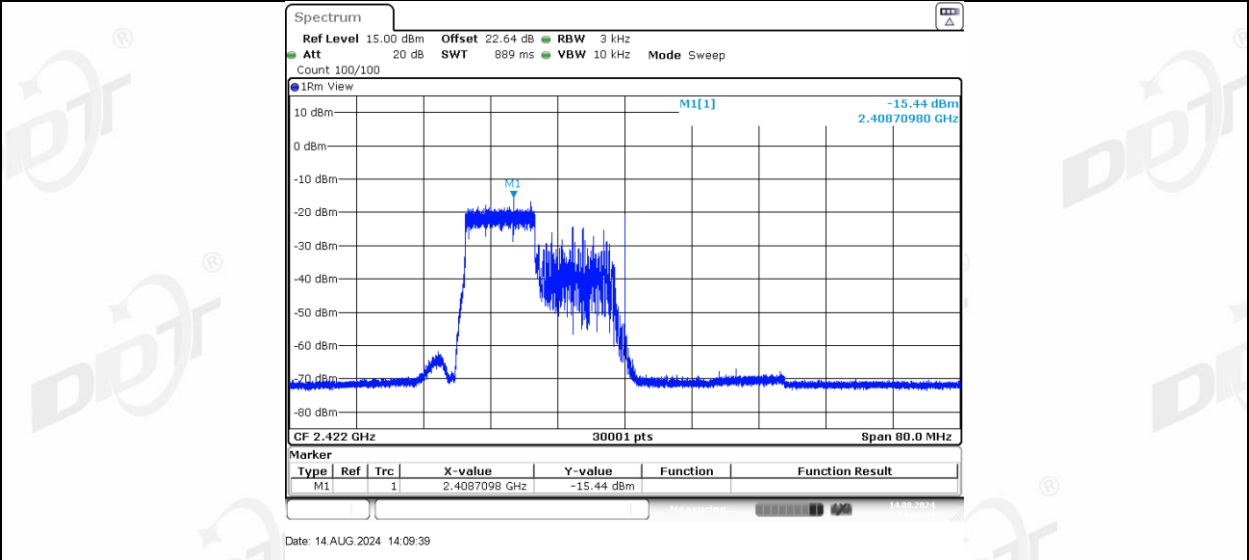
11AX40MIMO_Ant-3_2422_106Tone_RU56
