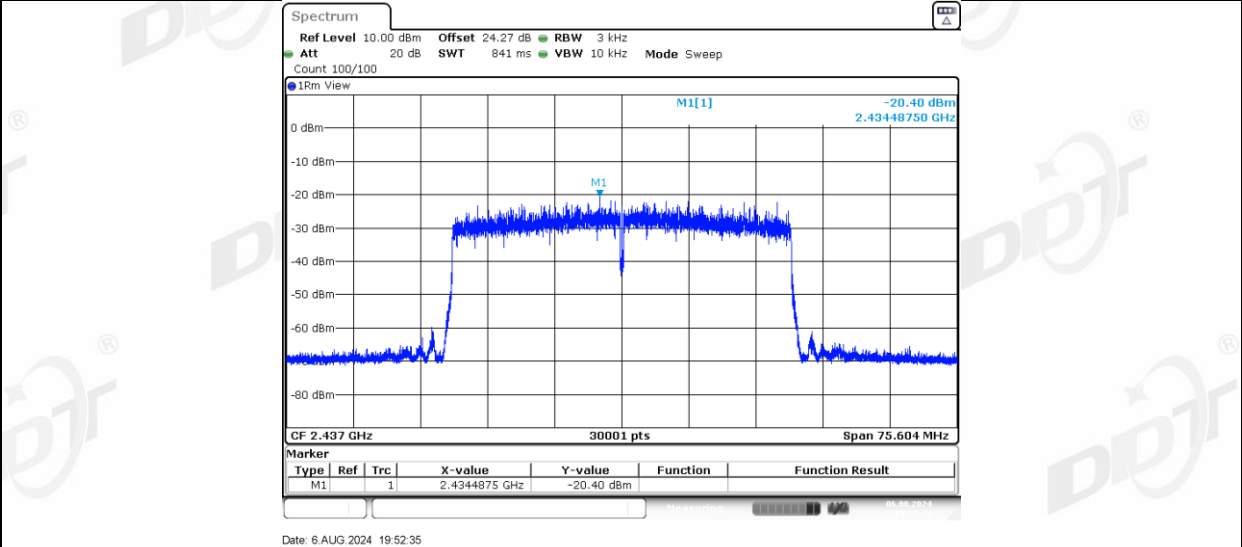
11AX40MIMO_Ant-3_2437
