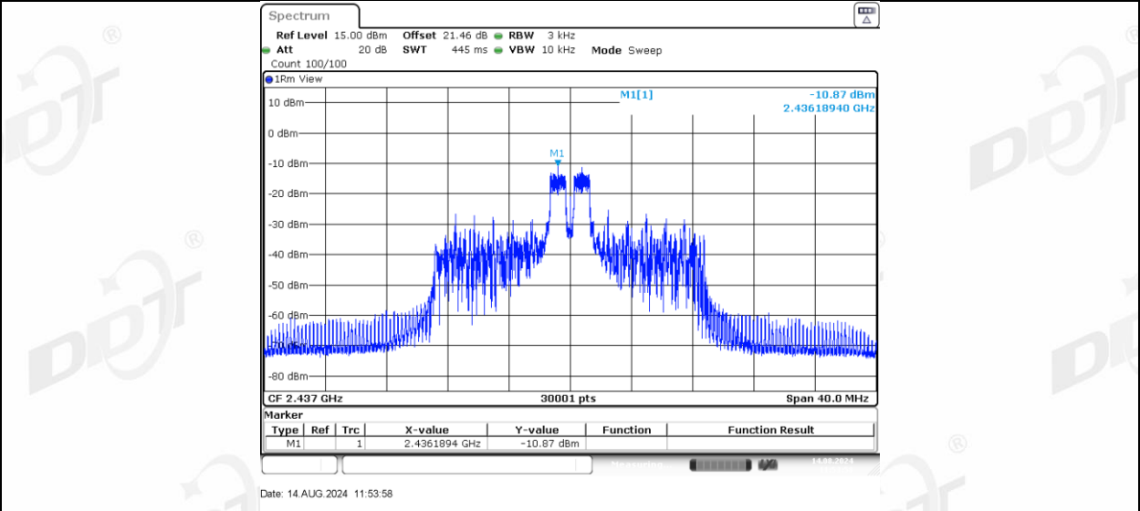
11AX20MIMO Ant-3 2437 26Tone RU8
