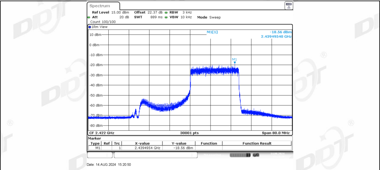
11AX40MIMO_Ant-3_2422_106Tone_RU53
