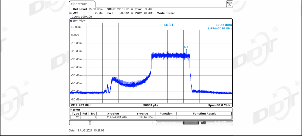
11AX40MIMO_Ant-3_2437_106Tone_RU53
