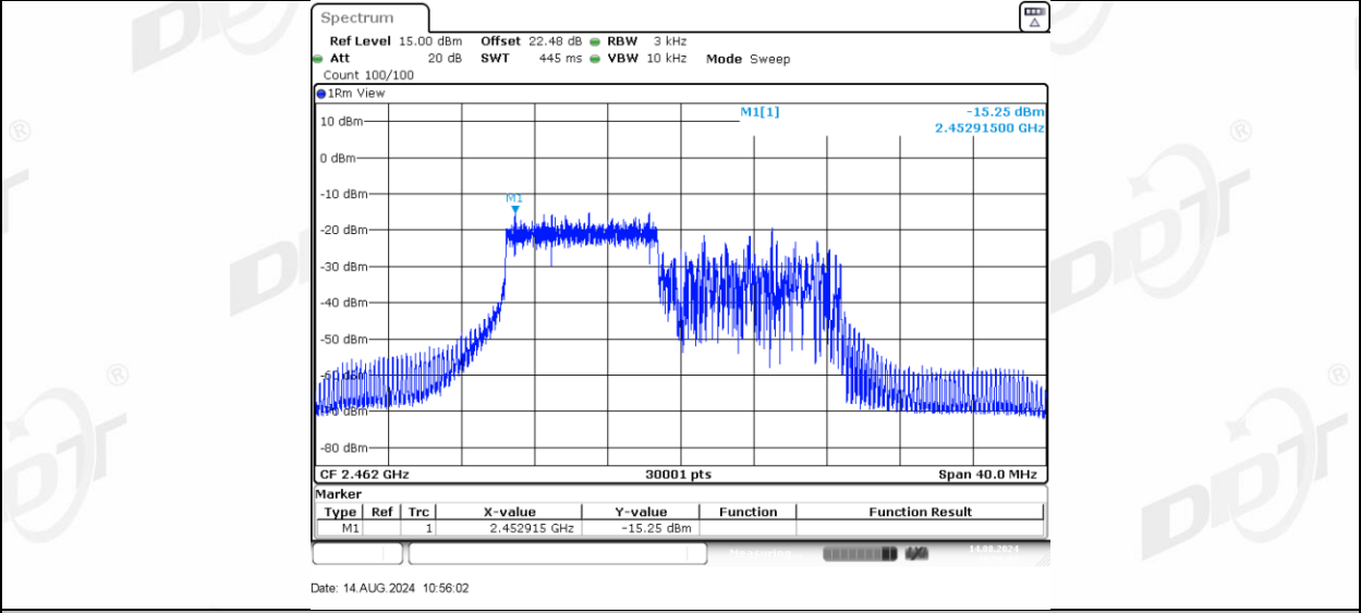
11AX20MIMO_Ant-1_2462_106Tone_RU54
