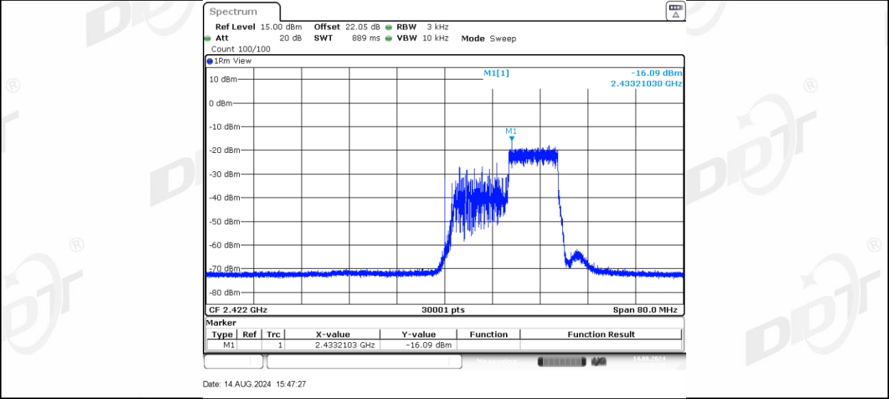
11AX40MIMO_Ant-3_2422_242Tone_RU61
