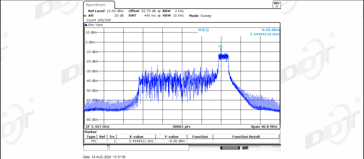
11AX20MIMO Ant-3 2437 52Tone RU37
