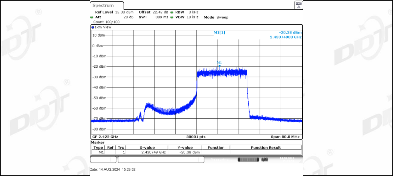
11AX40MIMO_Ant-1_2437_106Tone_RU53
