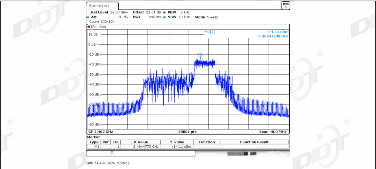
11AX20MIMO_Ant-1_2462_52Tone_RU40
