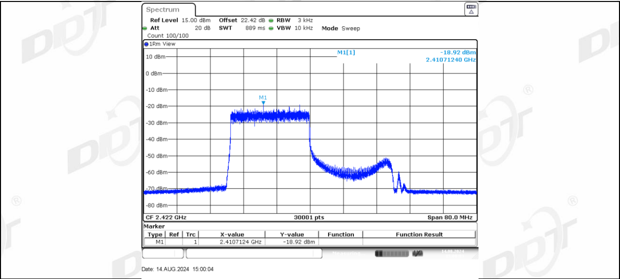
11AX40MIMO_Ant-3_2422_242Tone_RU62
