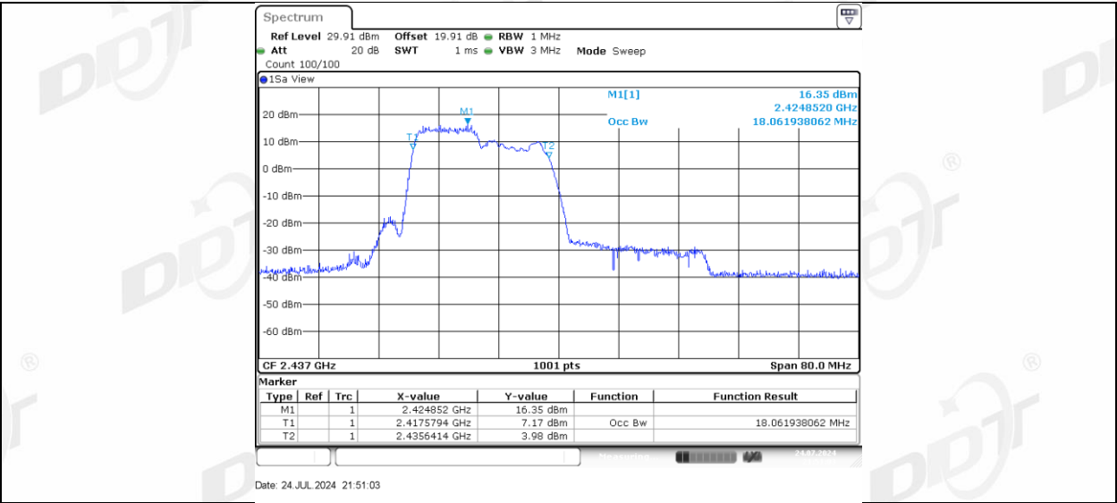
11AX40MIMO_Ant-3_2437_106Tone_RU56
