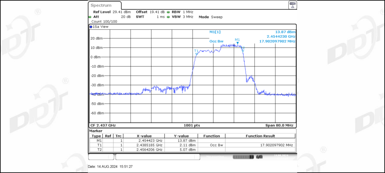
11AX40MIMO_Ant-3_2437_242Tone_RU61
