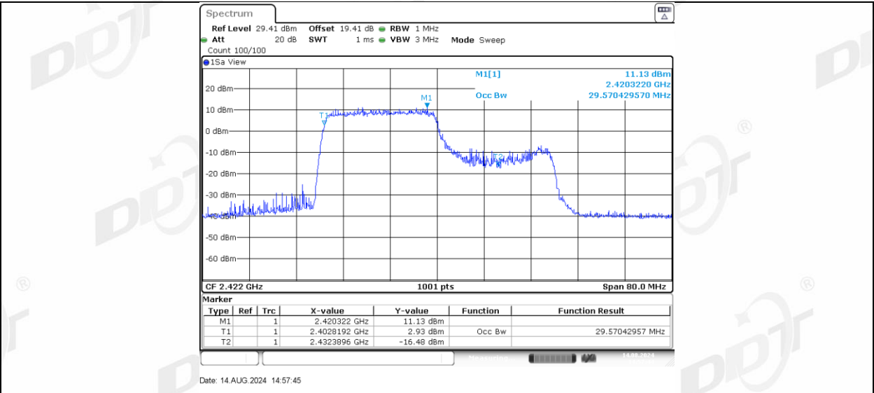
11AX40MIMO_Ant-3_2422_242Tone_RU62
