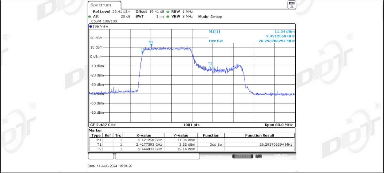
11AX40MIMO_Ant-3_2437_242Tone_RU62
