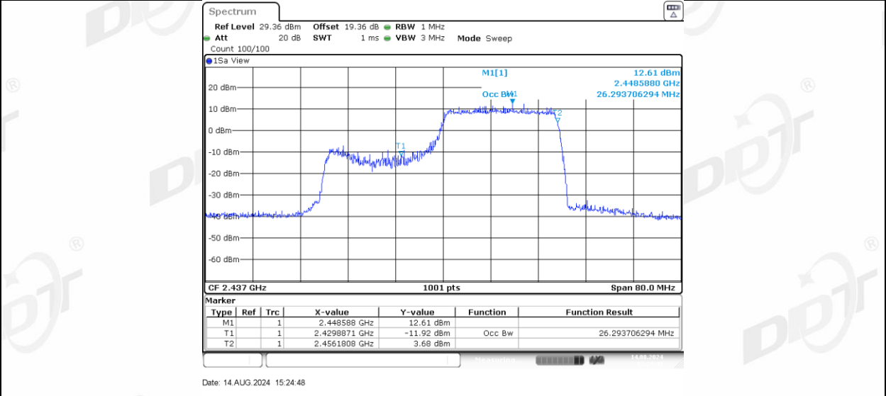
11AX40MIMO_Ant-3_2437_106Tone_RU53
