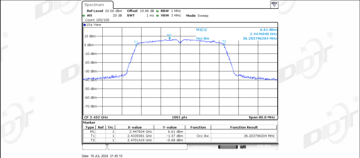
11N40MIMO_Ant-3_2452
