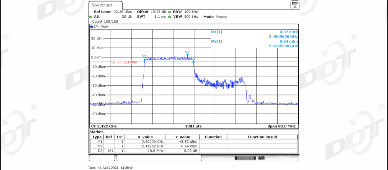
11AX40MIMO_Ant-1_2422_242Tone_RU62
