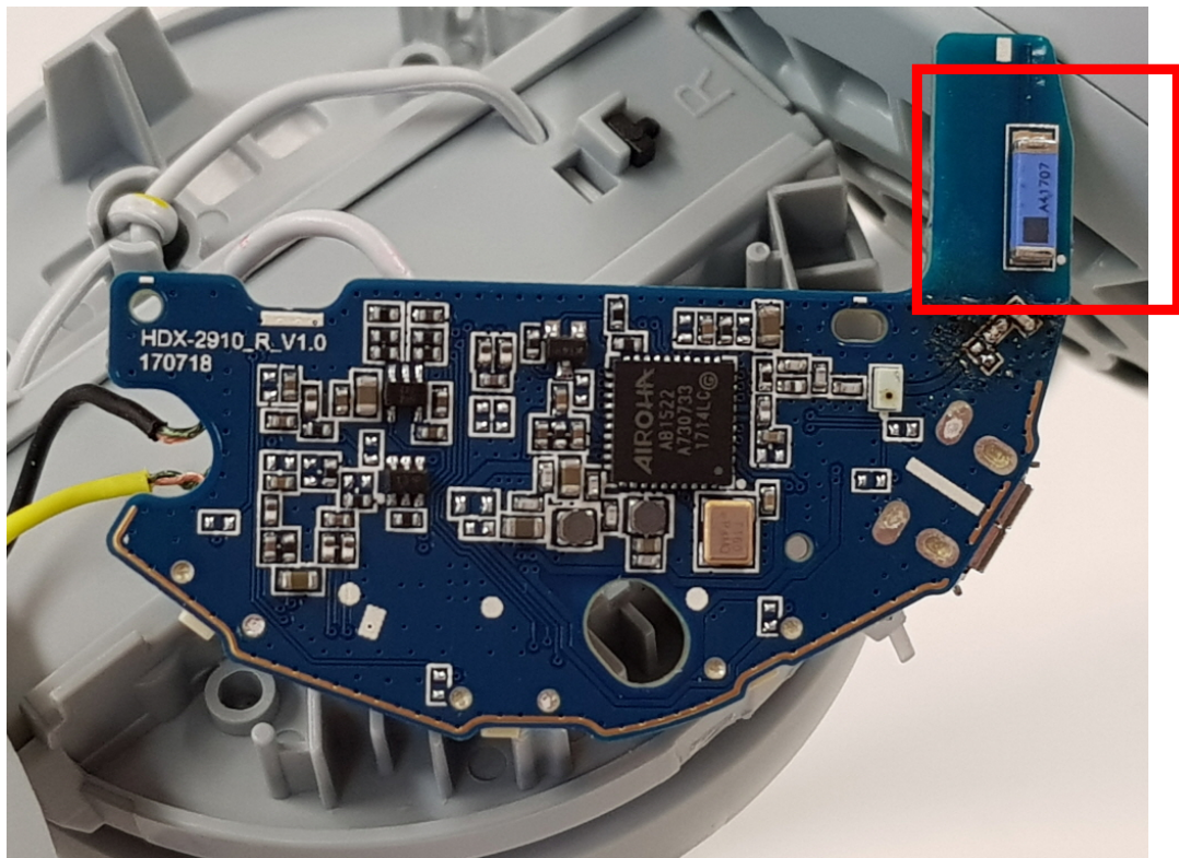
Antenna
