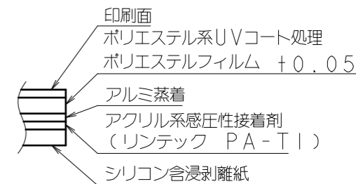
材料構成図
