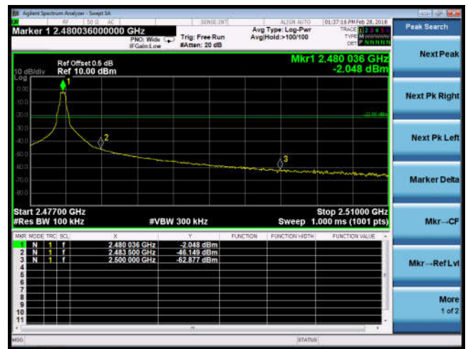
2480MHz(2.4GHz – 2.5GHz)
