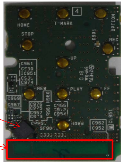
KEY_BT PWB
