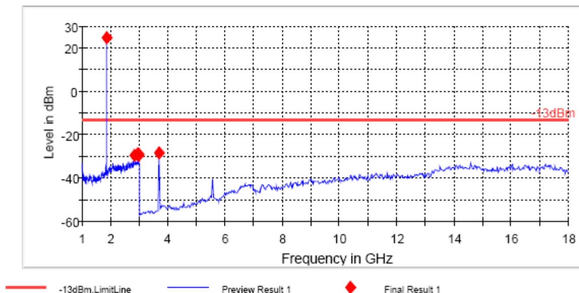
FCC 24 1-18GHz
