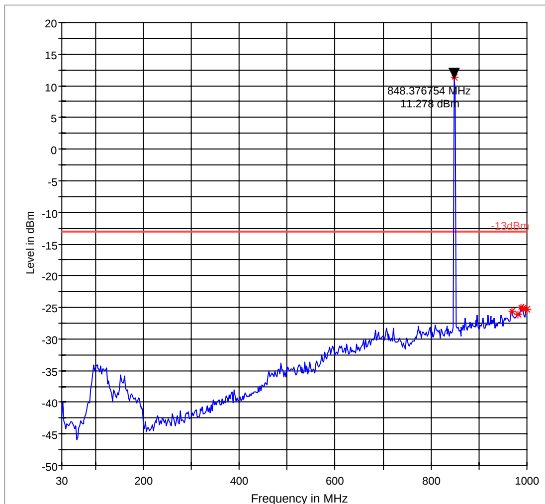
FCC 22 30-1000MHz
