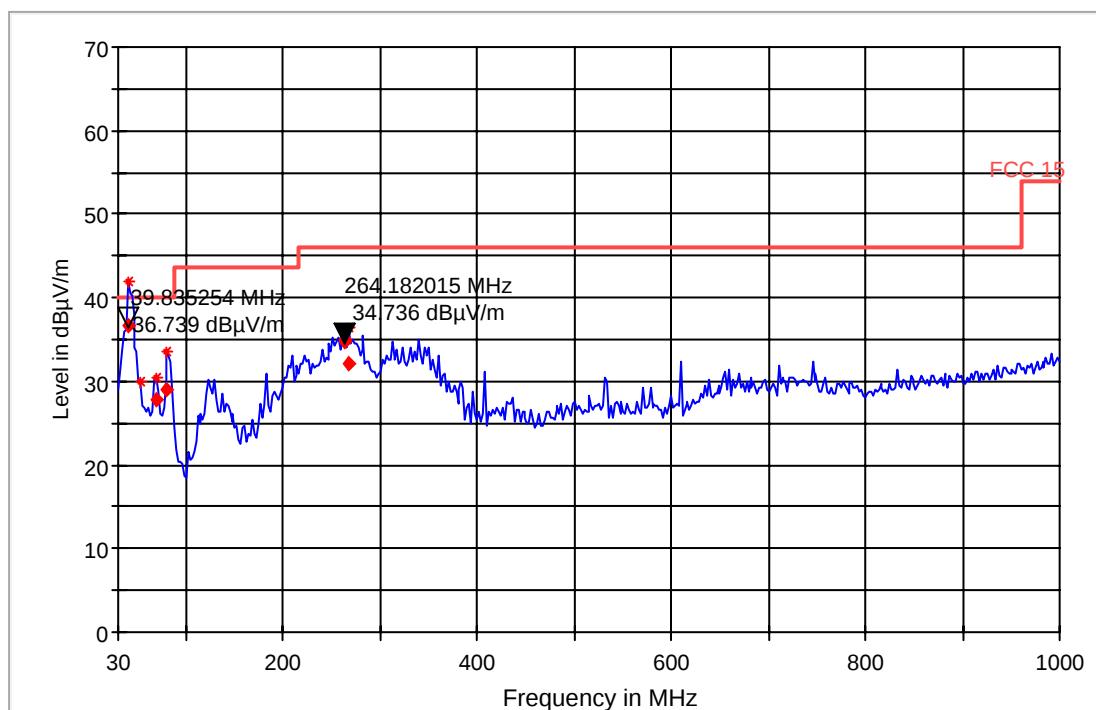
FCC 15 30-1000MHz
