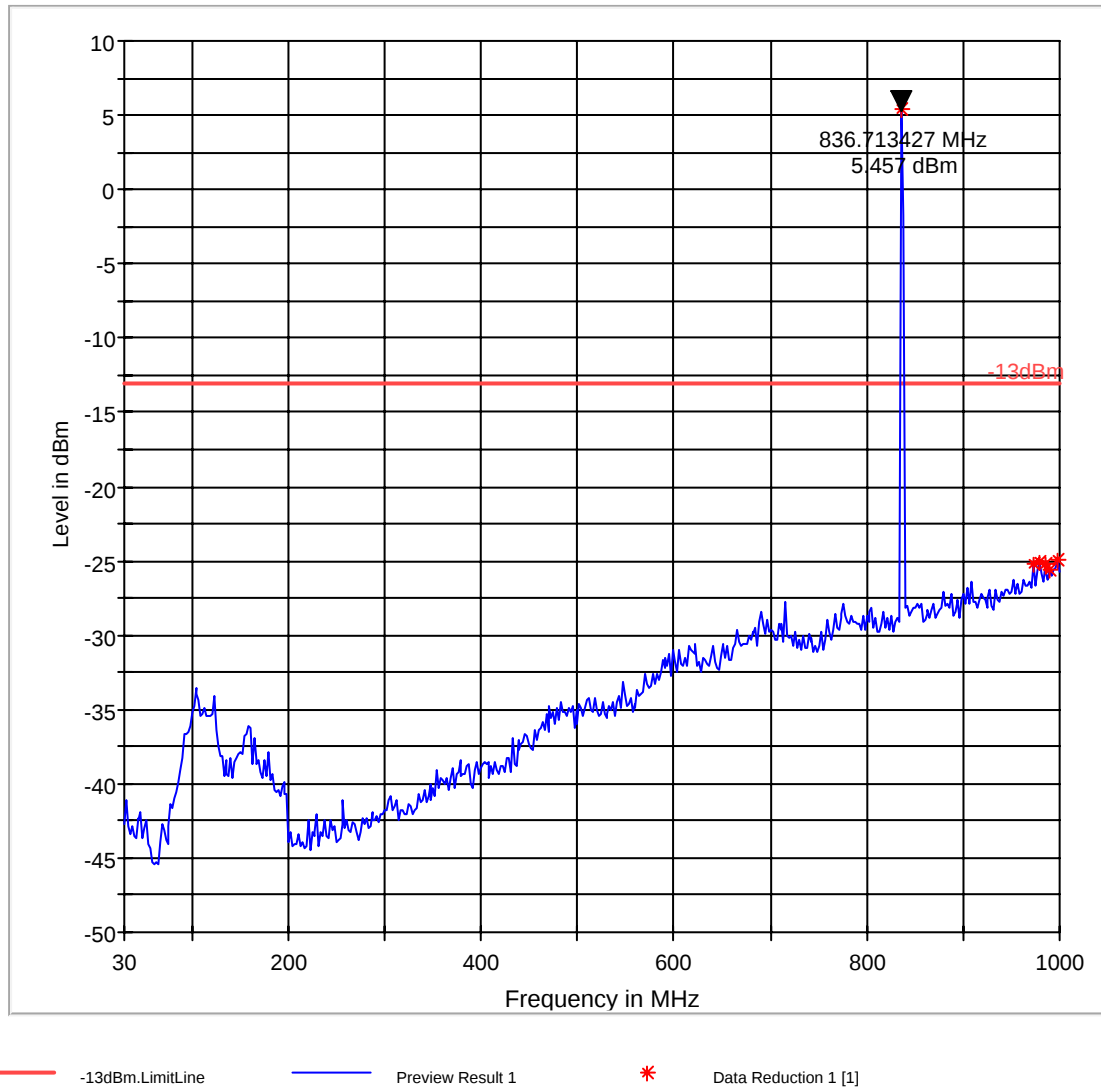
FCC 22 30-1000MHz
