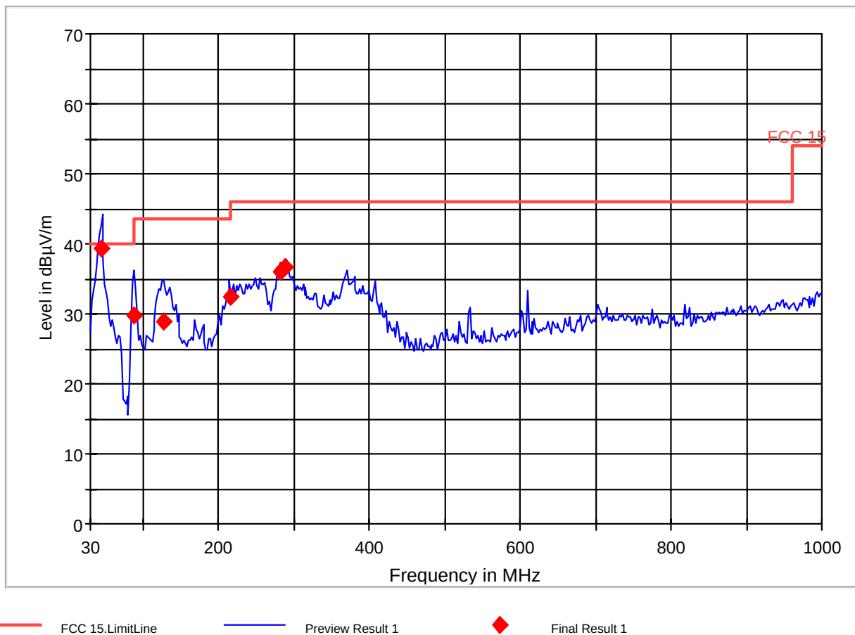
FCC 15 30-1000MHz
