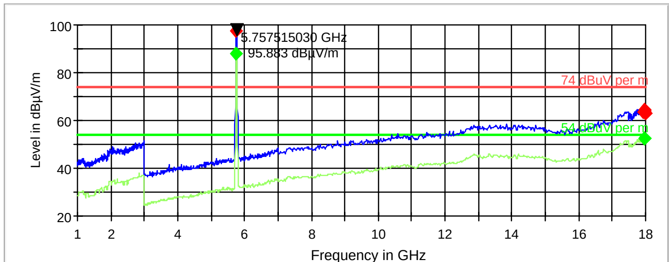
FCC 15 1-18GHz
