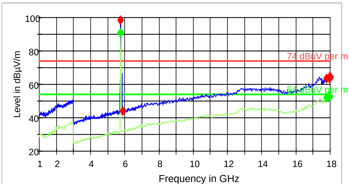
FCC 15 1-18GHz
