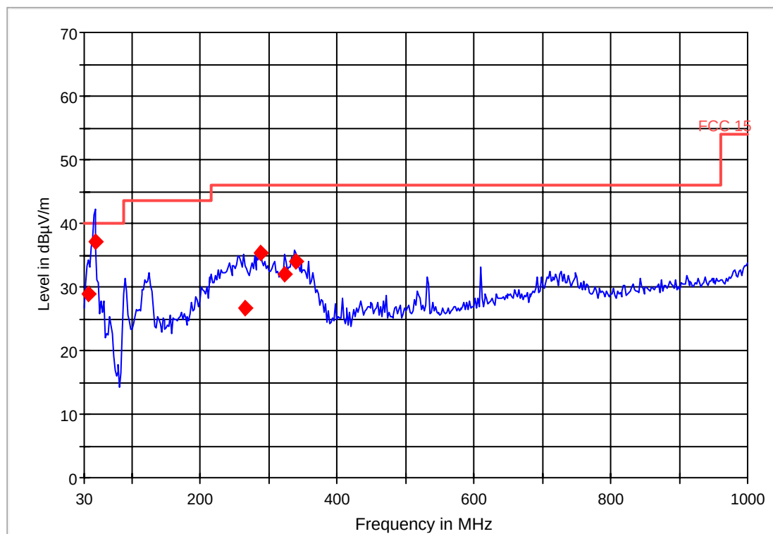
FCC 15 30-1000MHz
