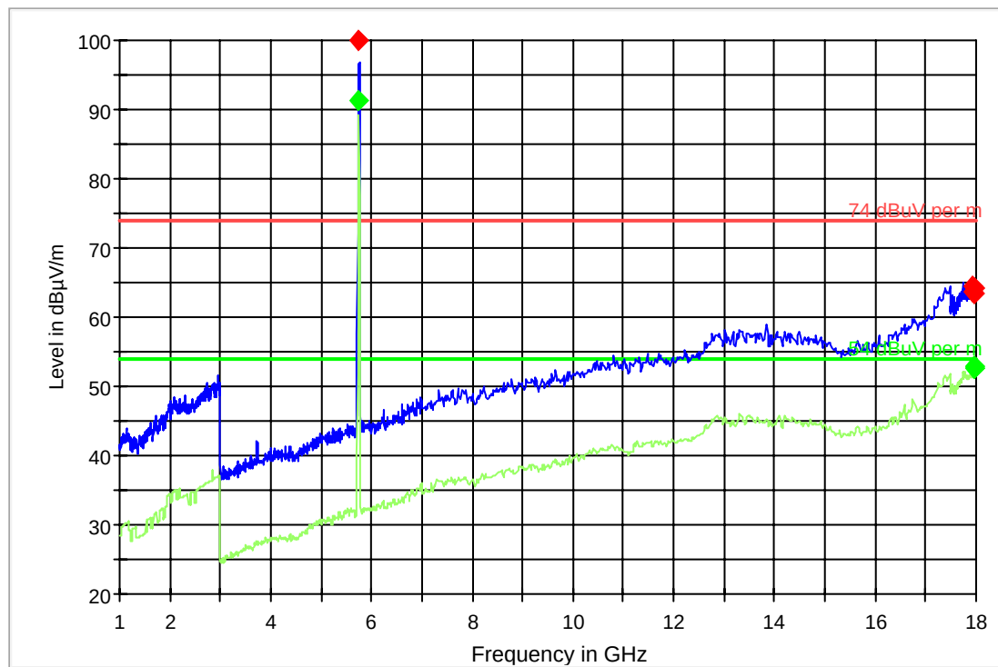
FCC 15 1-18GHz
