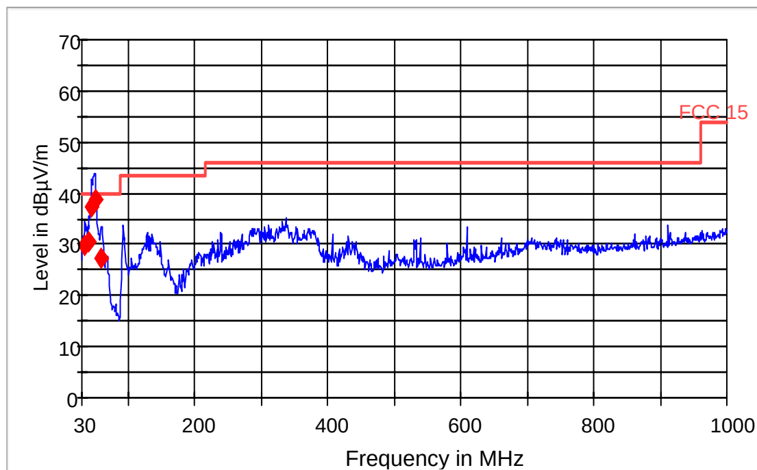
FCC 15 30-1000MHz
