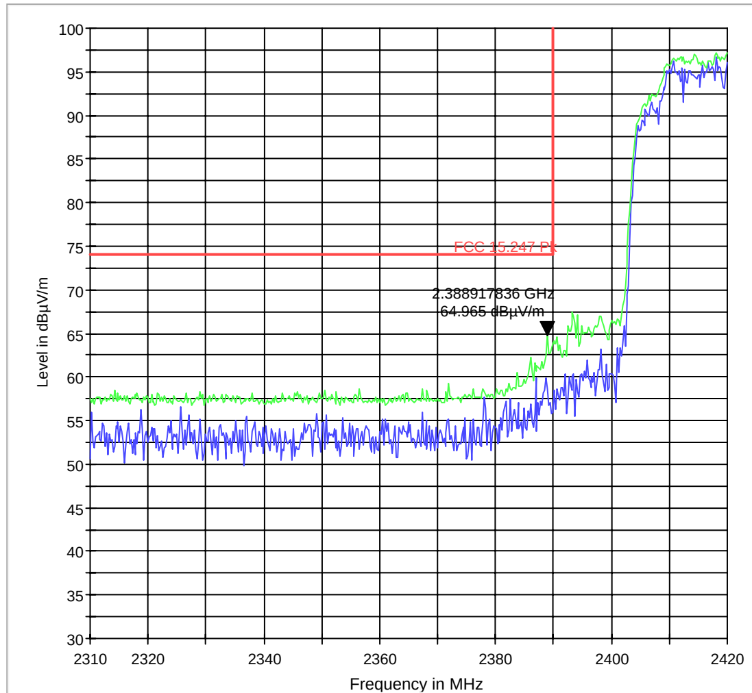
FCC 15.247 LBE Pk 3m
