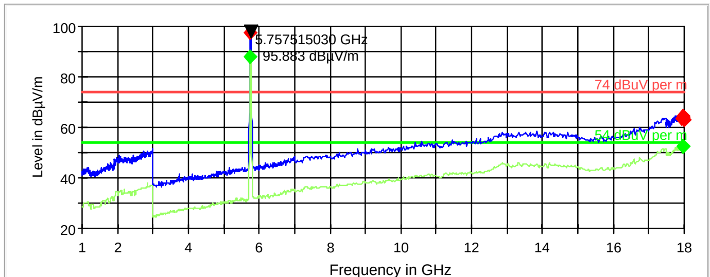
FCC 15 1-18GHz
