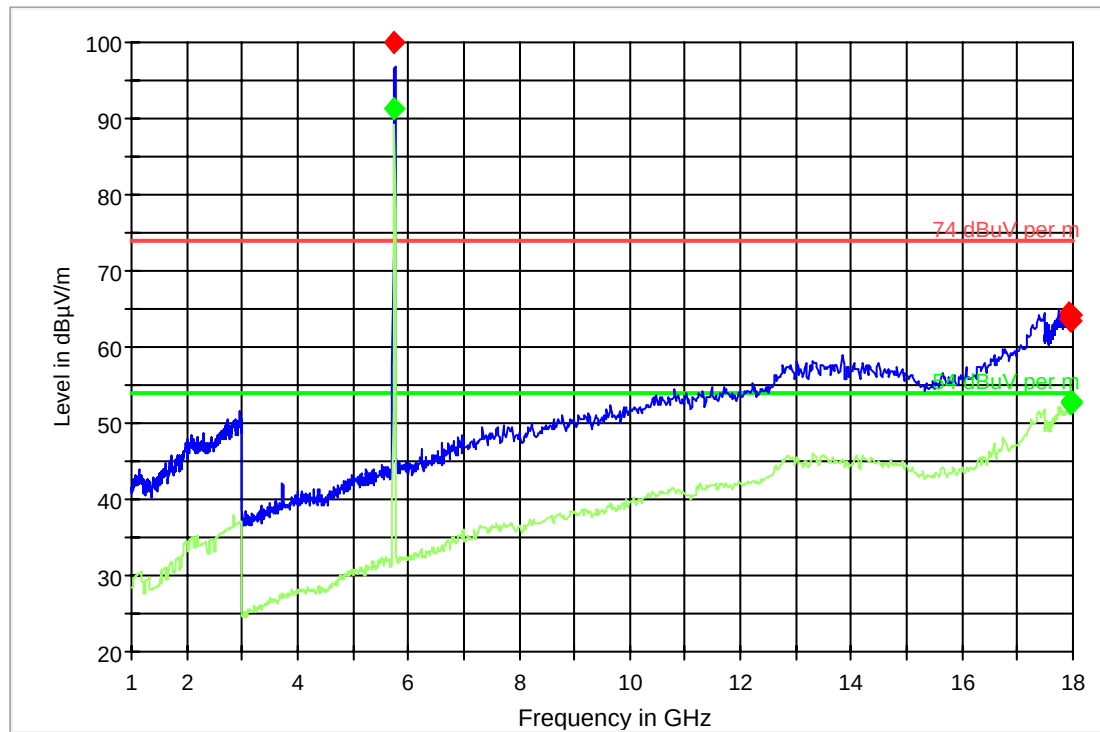
FCC 15 1-18GHz
