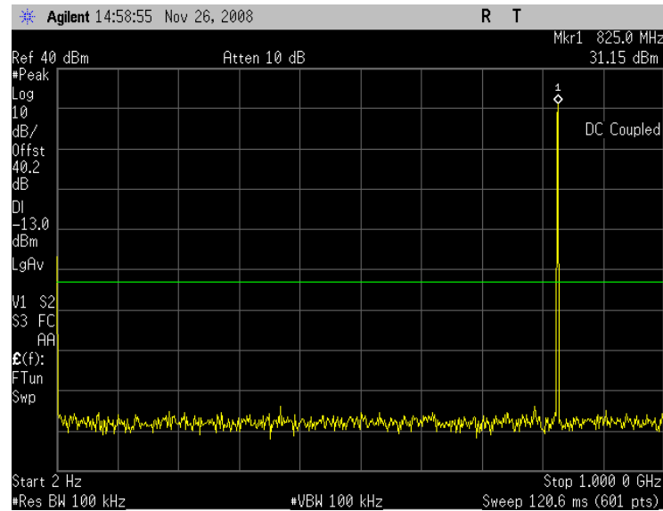
Plot 7.2 - 1 (GMSK Ch128)
