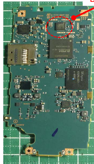
PWB IC side
