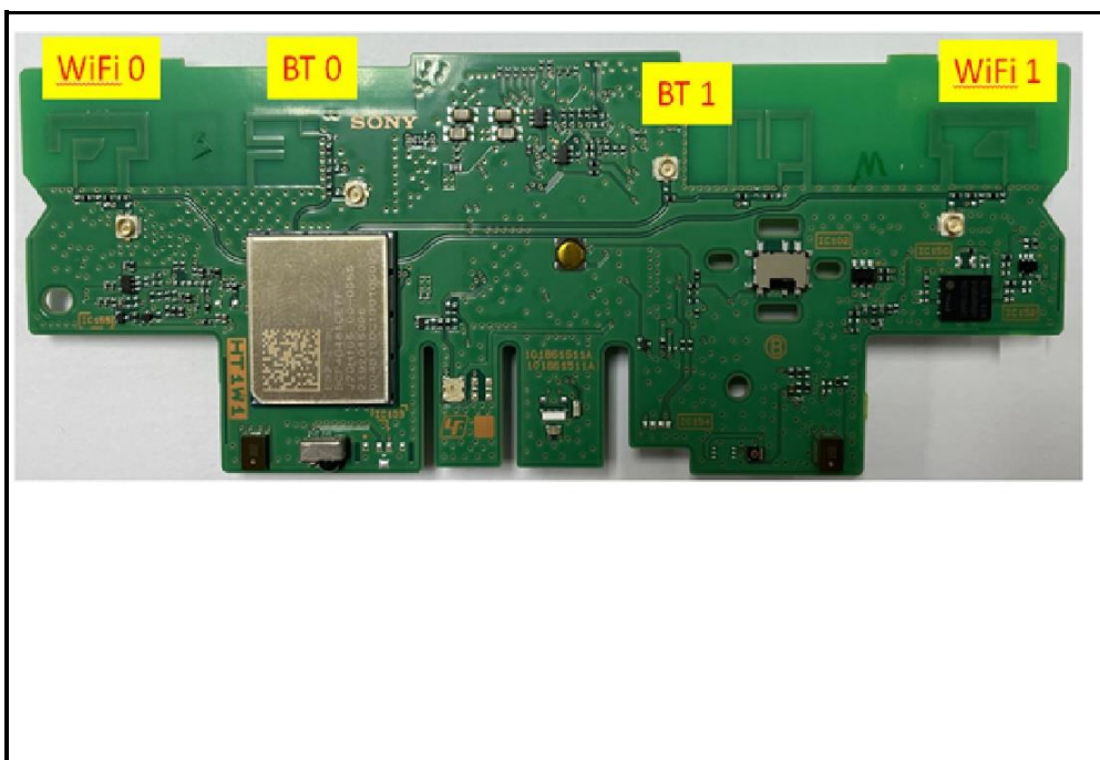
Antenna
