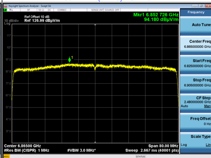
802.11ax (HE80) : CH 183
