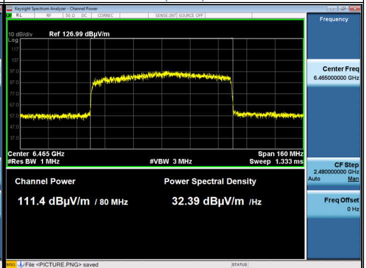
802.11ax (HE80) : CH 103
