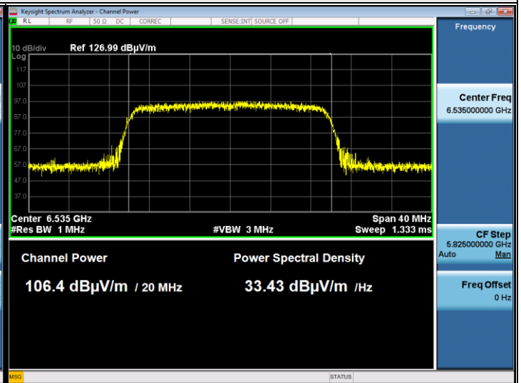
802.11ax (HE20) : CH 117
