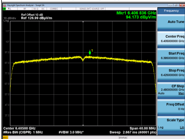
802.11ax (HE40) : CH 91
