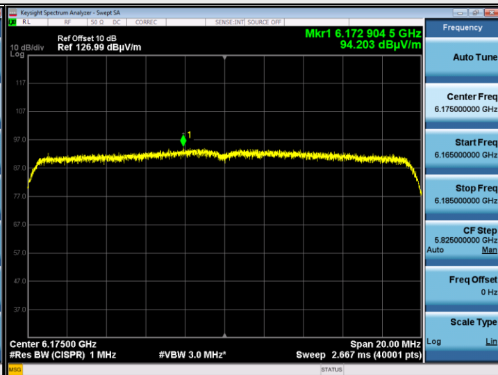
802.11ax (HE20) : CH 45
