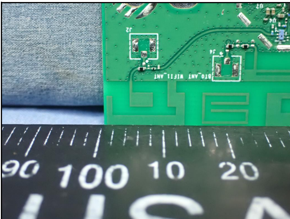
Antenna_Wifi 1
