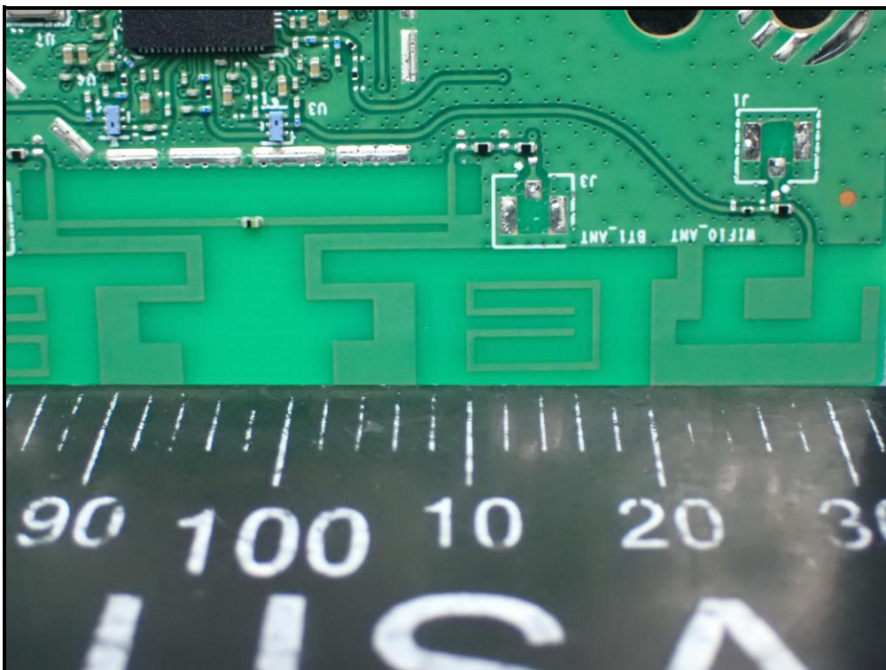
Antenna_BT 1
