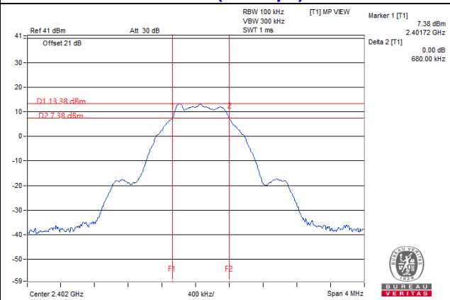
BT-LE Coded (500kbps) / CH 0
