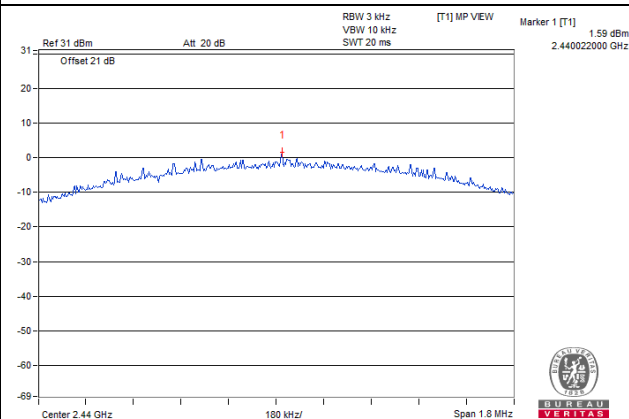
BT-LE Coded (500kbps) / CH 19
