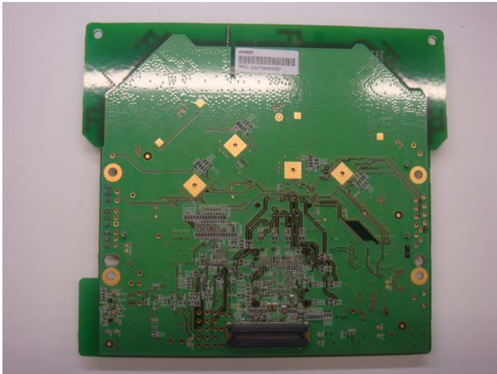
WHDI module Bottom
