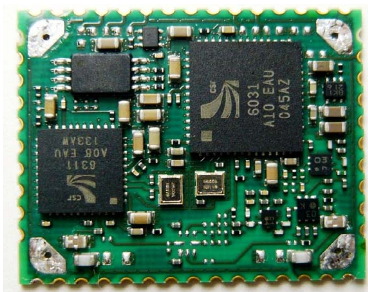
<半田付けを取り、シールド外した状態(without Shield)>
