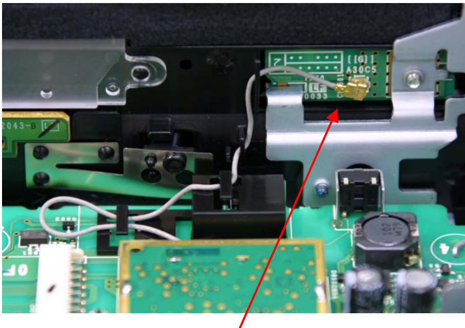
Antenna
