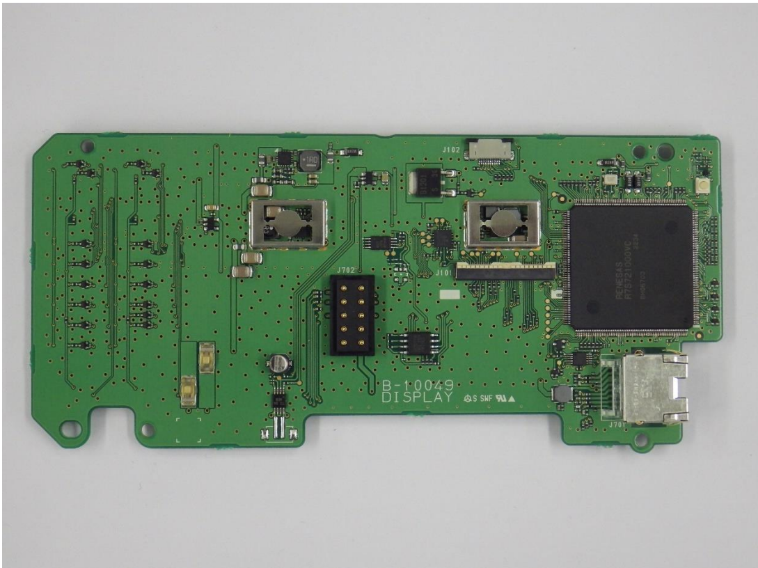
DISPLAY_sideB
