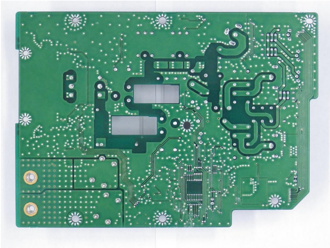
PA-G_sideB
