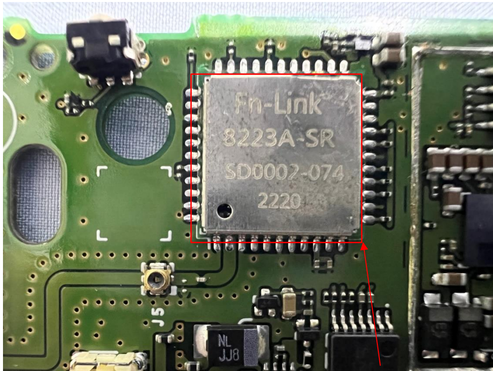
WIFI Module
