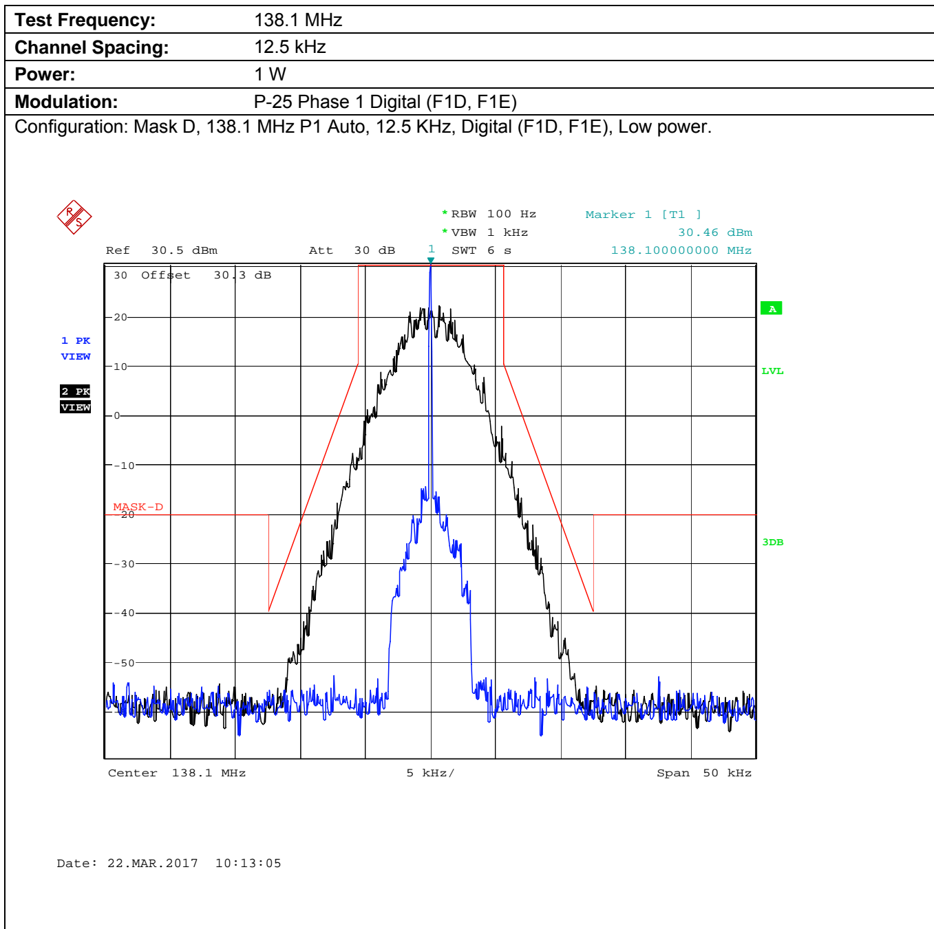
Plot 5.8.4.2.10. Emission Mask D, Low Power
