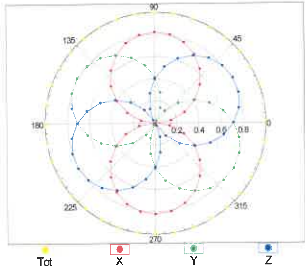
f=1800 MHz,R22
