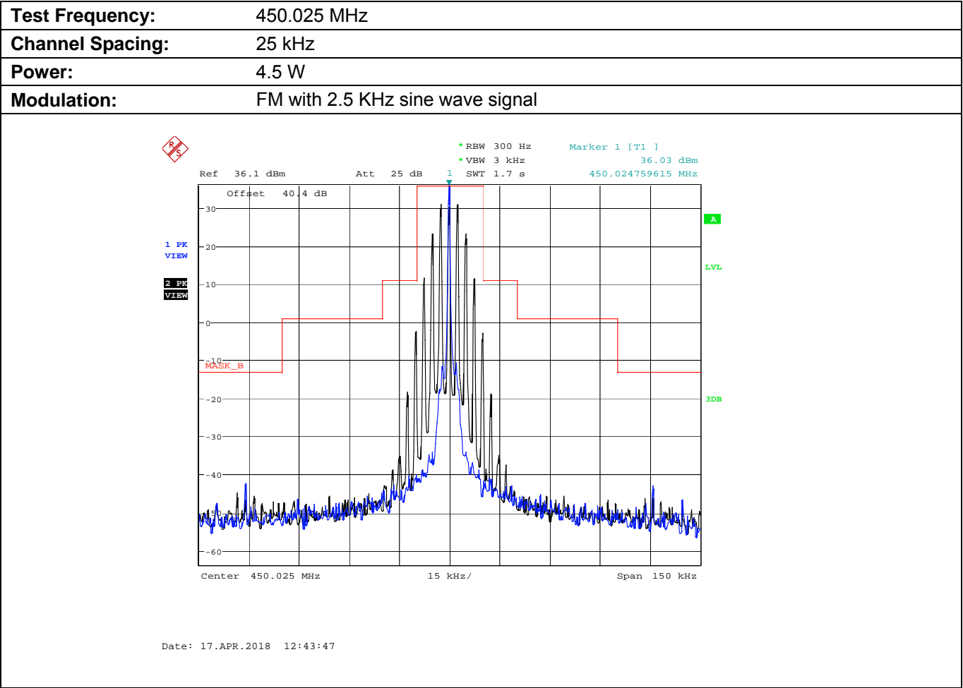
Plot 5.8.4.3.2. Emission Mask B, Low Power
