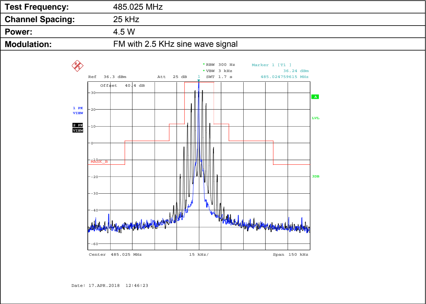
Plot 5.8.4.3.4. Emission Mask B, Low Power
