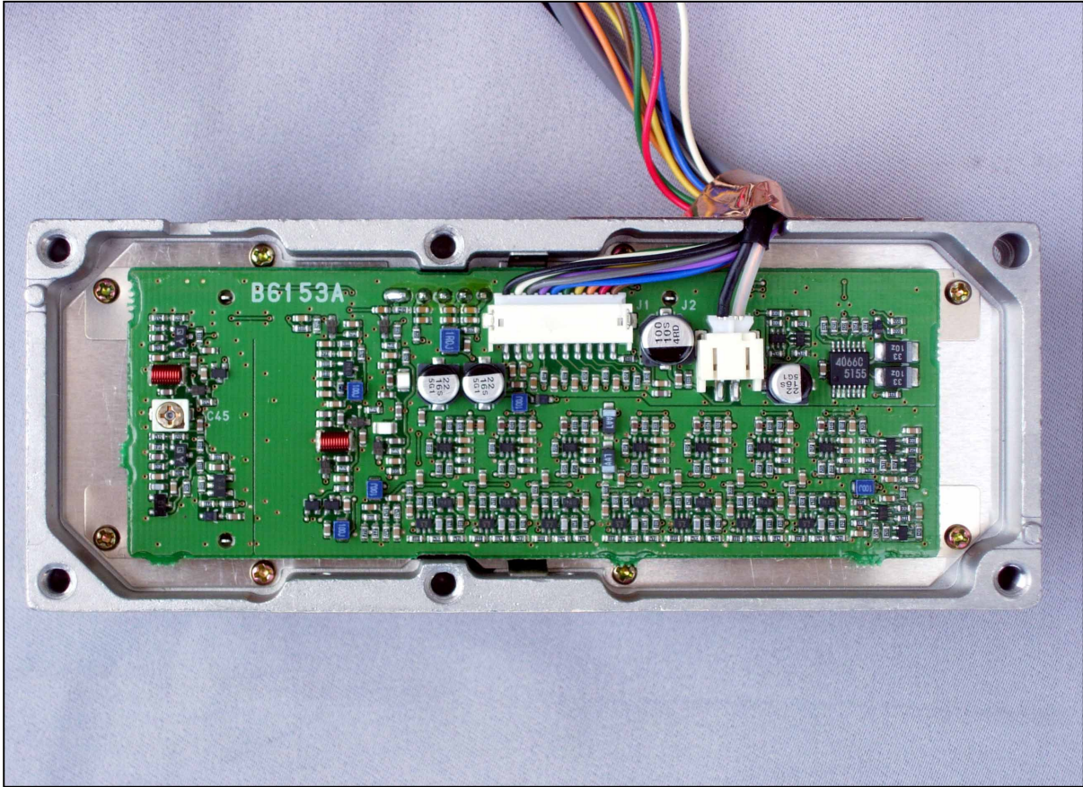
IF Unit
