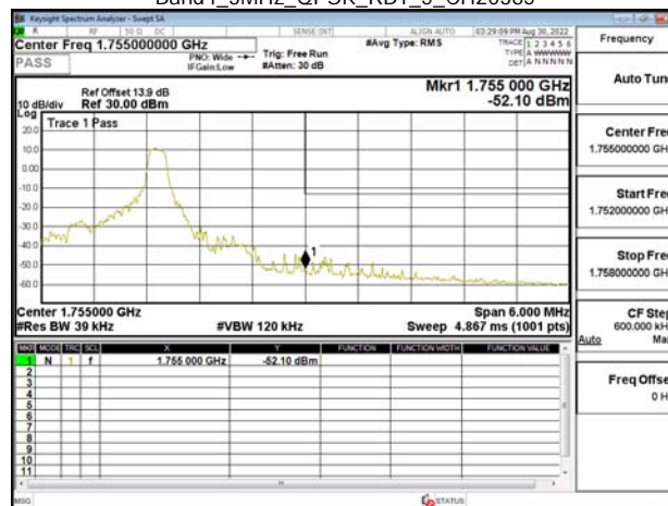
Band4_3MHz_QPSK_RB6_0_CH19965
