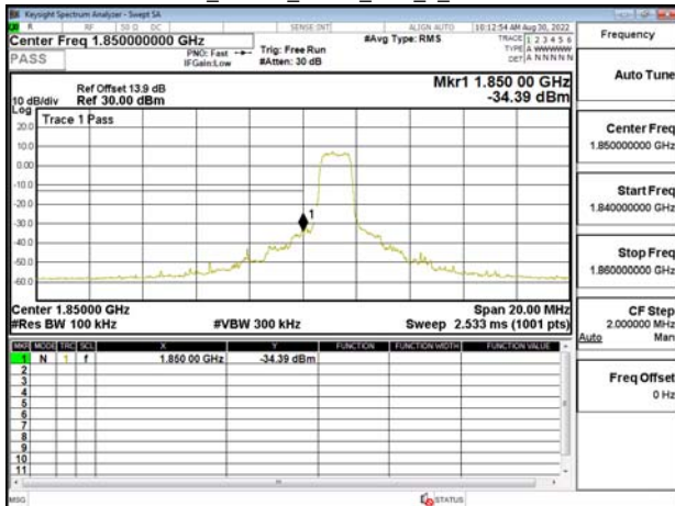
Band2_10MHz_QPSK_RB6_0_CH18650
