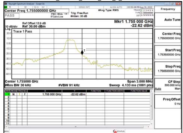
Band4_1.4MHz_QPSK_RB1_5_CH20393
