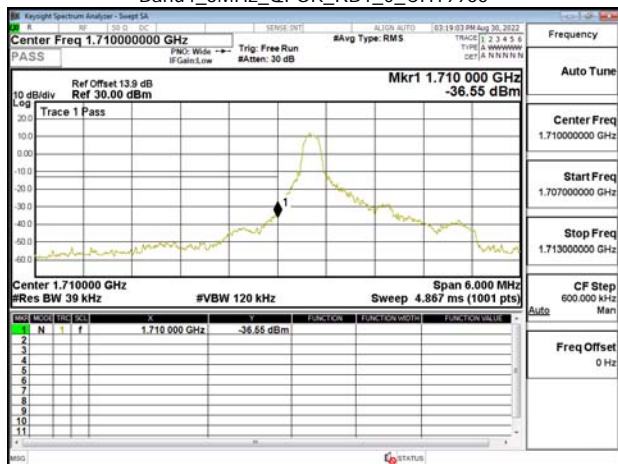
Band4_3MHz_QPSK_RB1_0_CH19965
