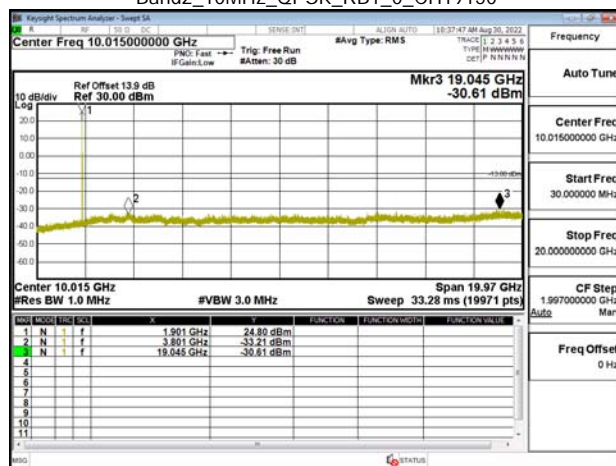
Band2_10MHz_QPSK_RB1_0_CH19150
