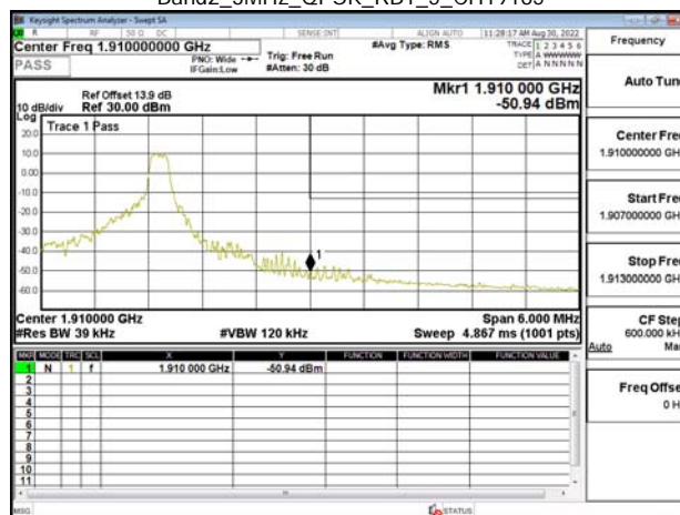
Band2_3MHz_QPSK_RB1_5_CH19185
