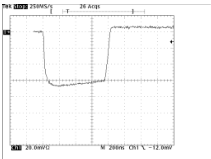
Fig. 3.2.3.4 Long Pulse (24 nm Range) Scale: 20 mV/div. 200 ns/div.
