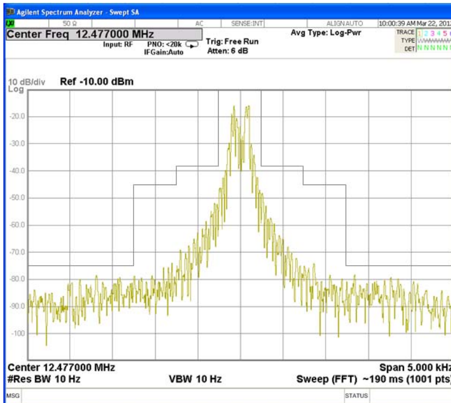
Fig. 3.3.26 NBDP(FEC): Tx Frequency 12477 kHz
