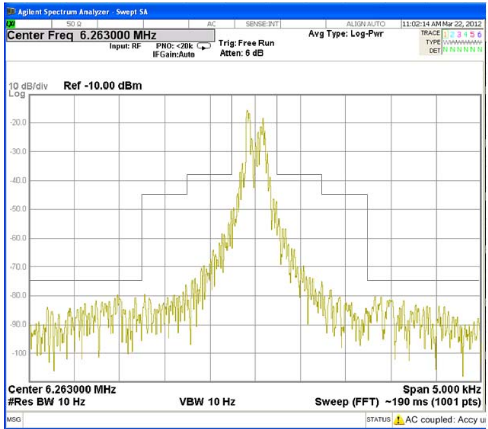
Fig. 3.3.24 NBDP(FEC): Tx Frequency 6263 kHz
