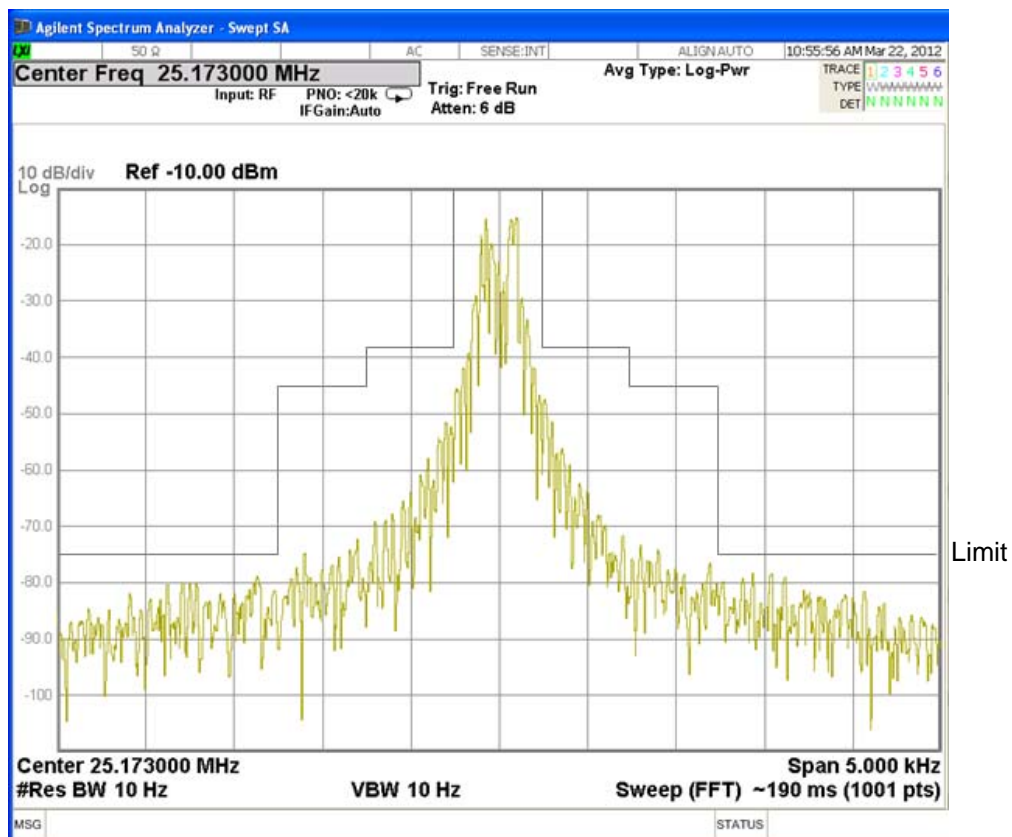
Fig. 3.4.21 NBDP(ARQ): Tx Frequency 25173 kHz
