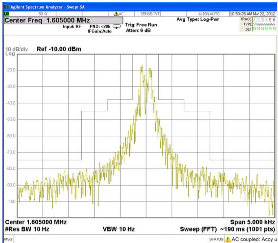
Fig. 3.3.22 NBDP(FEC): Tx Frequency 1605 kHz
