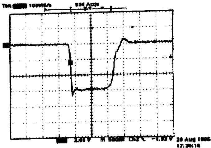
Scale: 2 kV/div. 500 ns/div.
