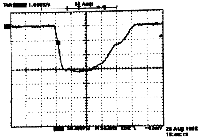
Scale: 50 mV/div. 50 ns/div.
