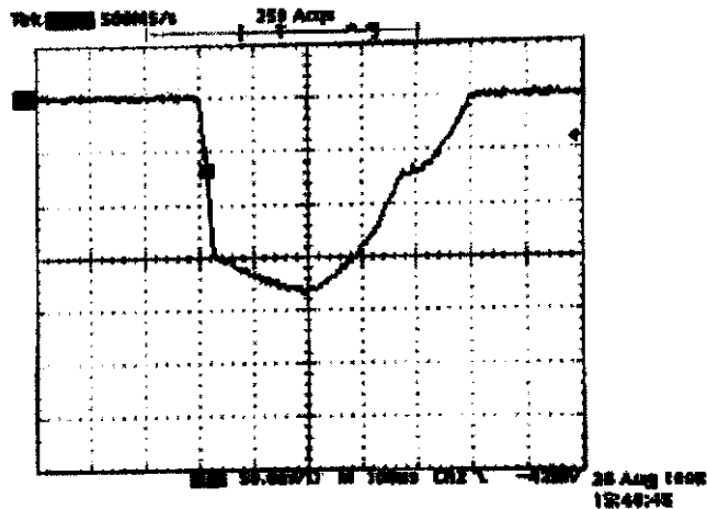
Scale: 50 mV/div. 100 ns/div.
