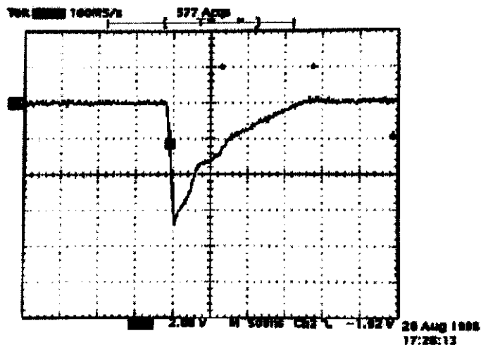
Scale: 2 kV/div. 500 ns/div.
