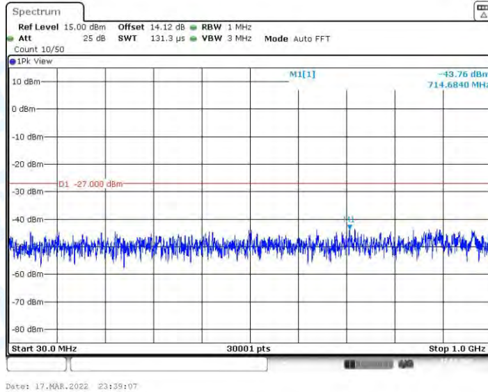
11N40MIMO_Ant1_5670_30~1000
