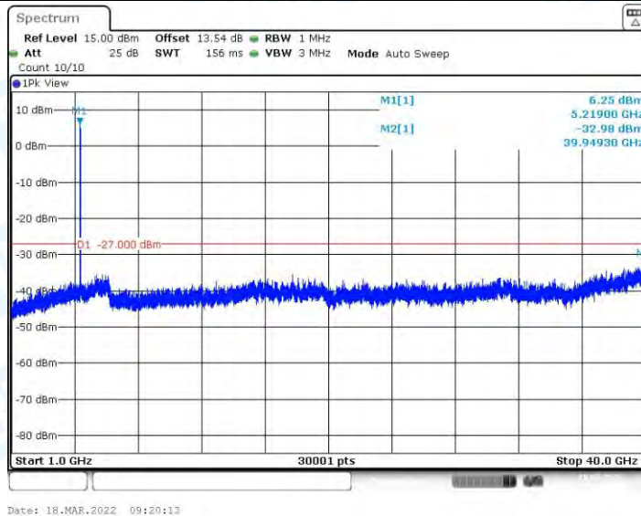
11AC20MIMO_Ant1_5220_1000~40000
