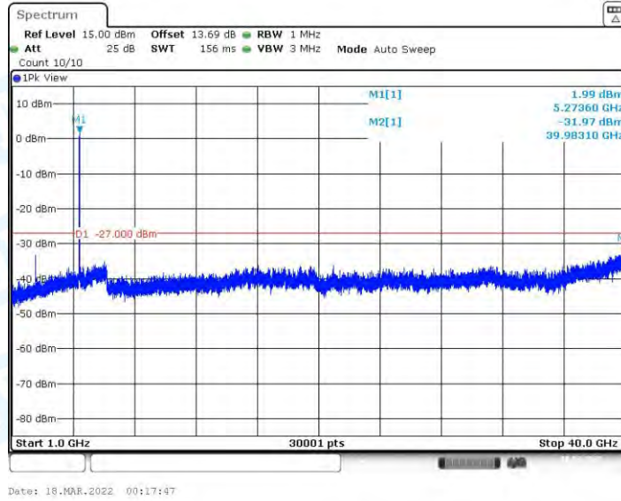
11AC40MIMO_Ant1_5270_1000~4000
