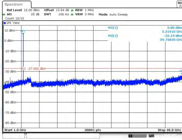
11AC20MIMO_Ant1_5320_1000~40000
