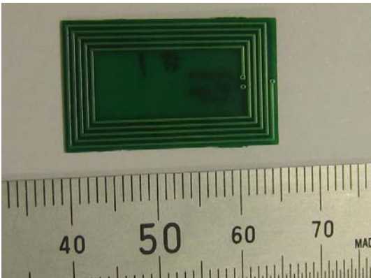
NFC PCB Back
