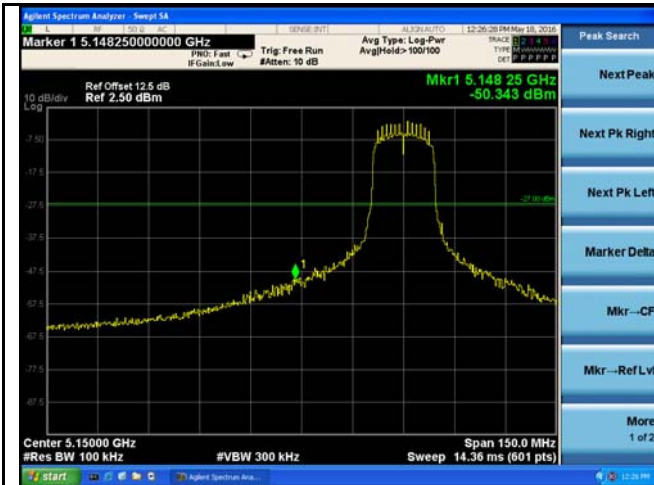
5150-5350MHz Band Edge - Low CH 5180
