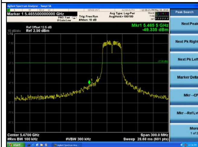
5470-5725MHz Band Edge - Low CH 5510
