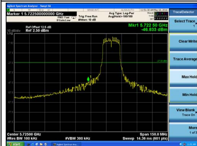
5725-5850MHz Band Edge - Low CH 5745
