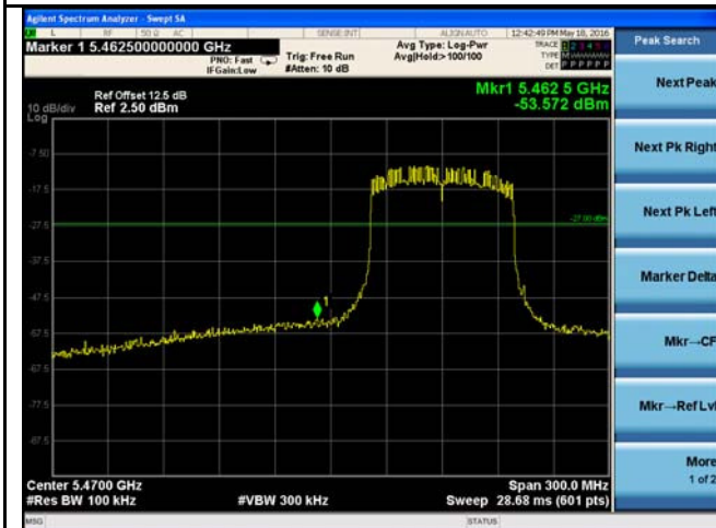
5470-5725MHz Band Edge - Low CH 5530
