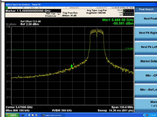
5470-5725MHz Band Edge - Low CH 5500
