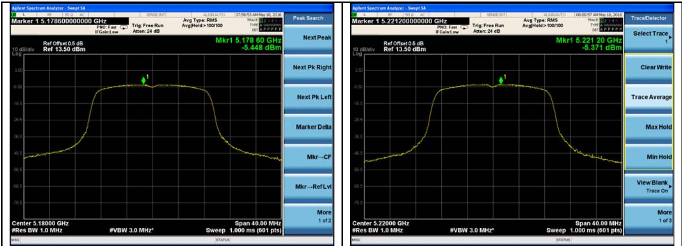
5150-5250MHz PSD - Low CH 5180
