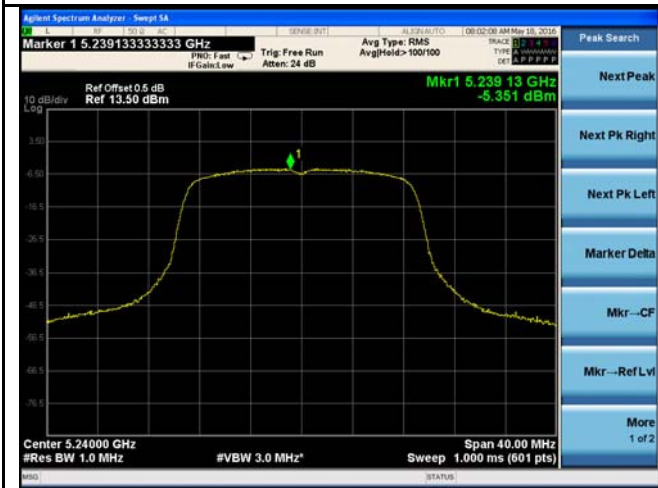
5150-5250MHz PSD - High CH 5240
