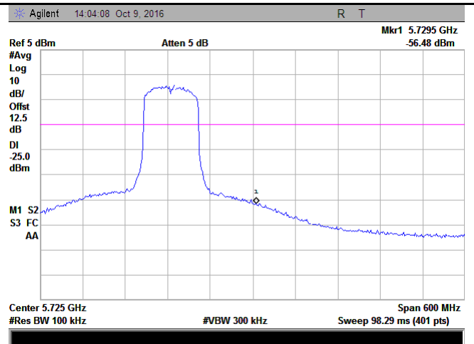
5470-5725MHz Band Edge - High CH 5610
