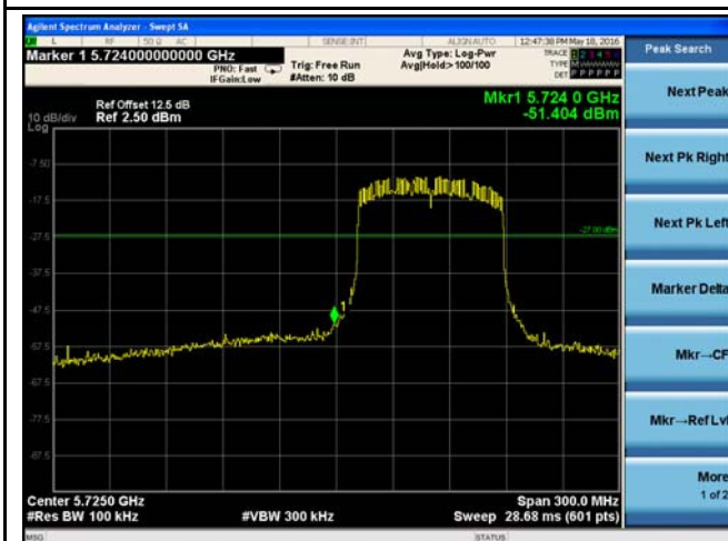
5725-5850MHz Band Edge - Low CH 5775
