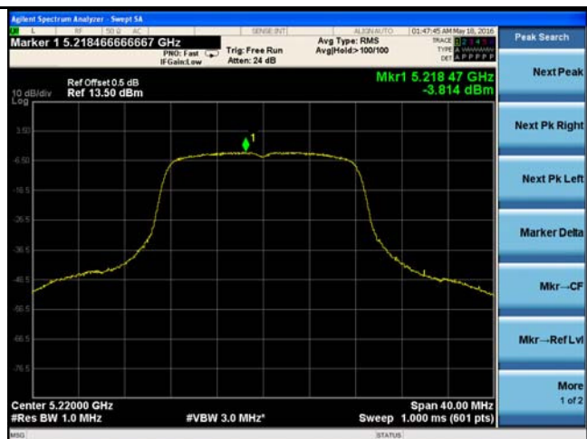
5150-5250MHz PSD - Middle CH 5220
