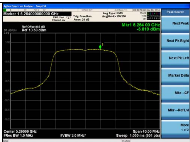
5250-5350MHz PSD - Low CH 5260
