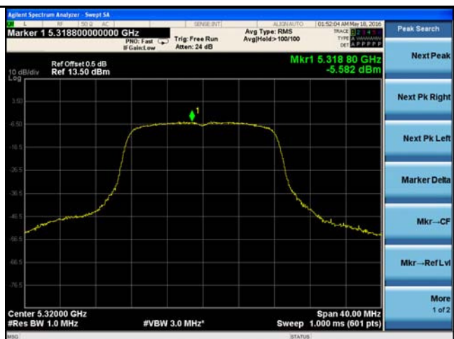
5250-5350MHz PSD - High CH 5320
