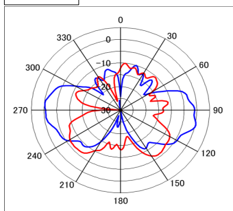
3700MHz Red:Vertical
