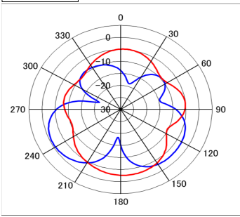
698MHz Red:Vertical
