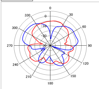
2500MHz Red:Vertical
