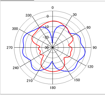
1710MHz(B4/B66) Red:Vertical
