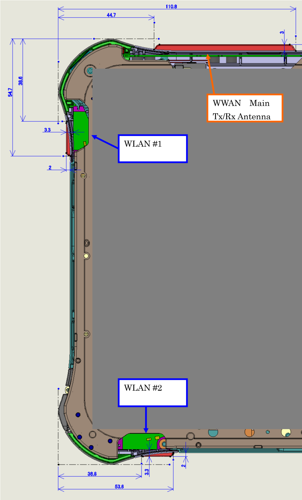
3_2) Diagram: Antenna spacer Unit: mm
