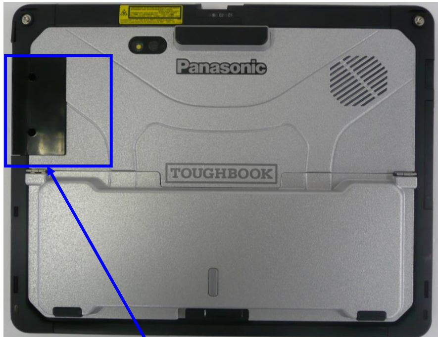
HF-RFID Module
