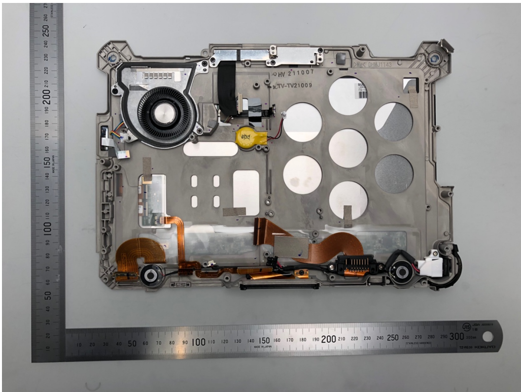
LCD module - Back
