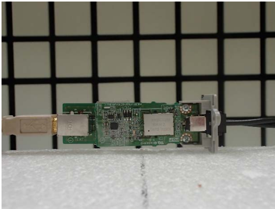
Module Z-axis
