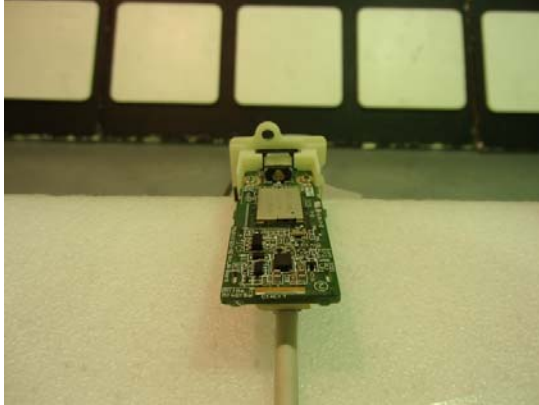
Module Y-axis
