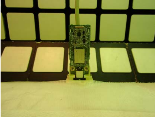
Module Z-axis
