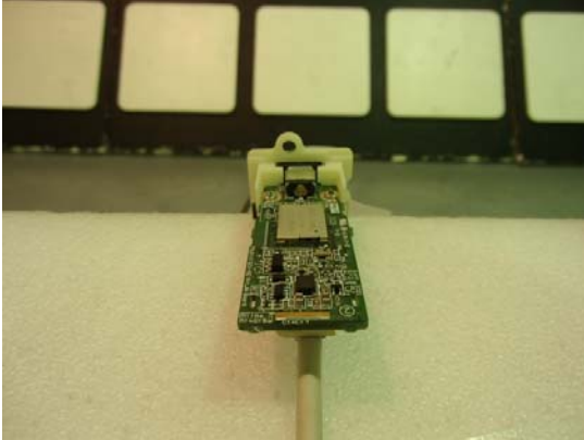
Module Y-axis
