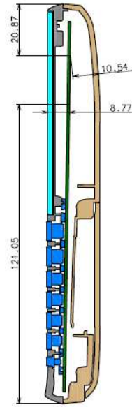
Sec. D-D (Pattern antenna)
