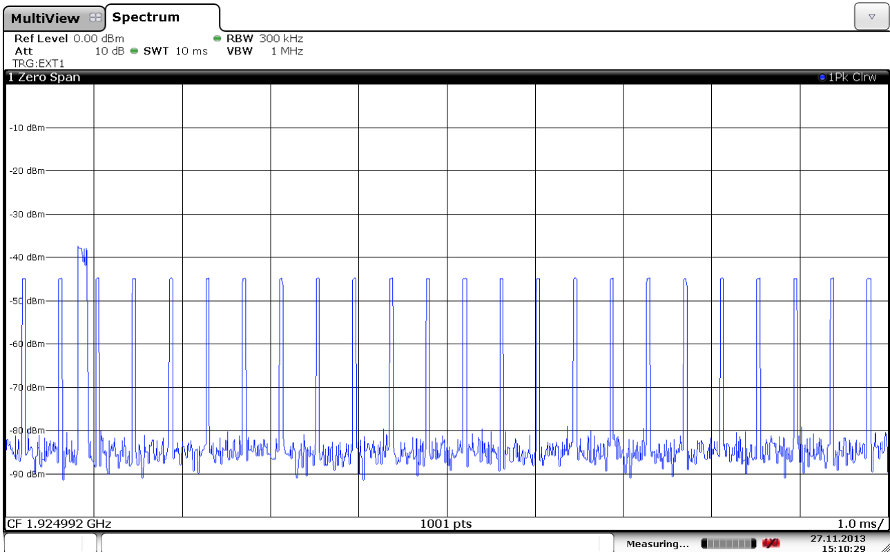
35 µs Pulses
