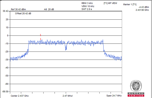
802.11g : CH6
