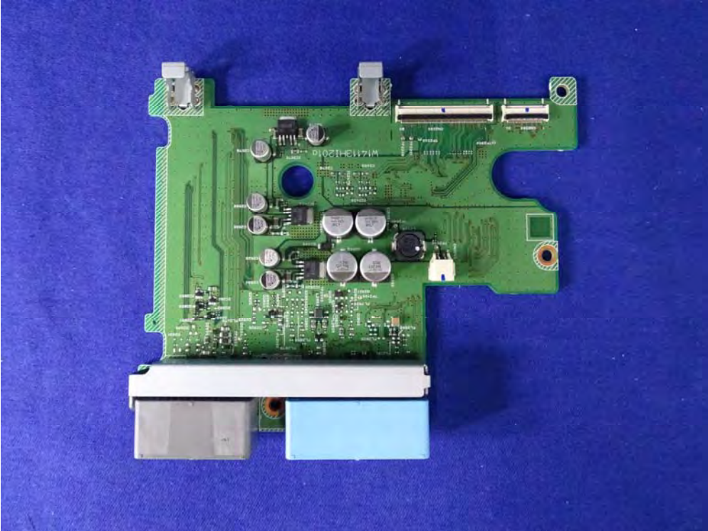
(59) EUT Photo
