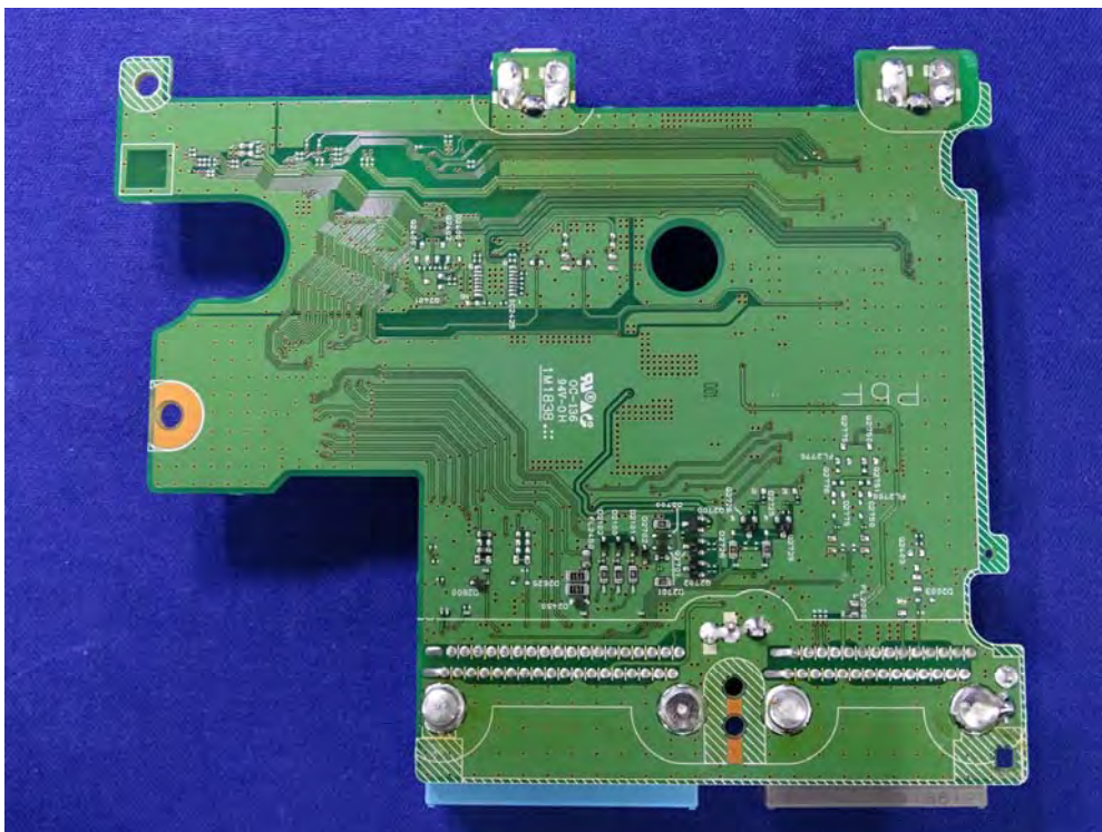
(61) EUT Photo
