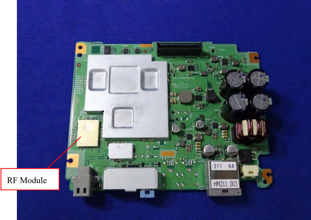
(17) EUT Photo
