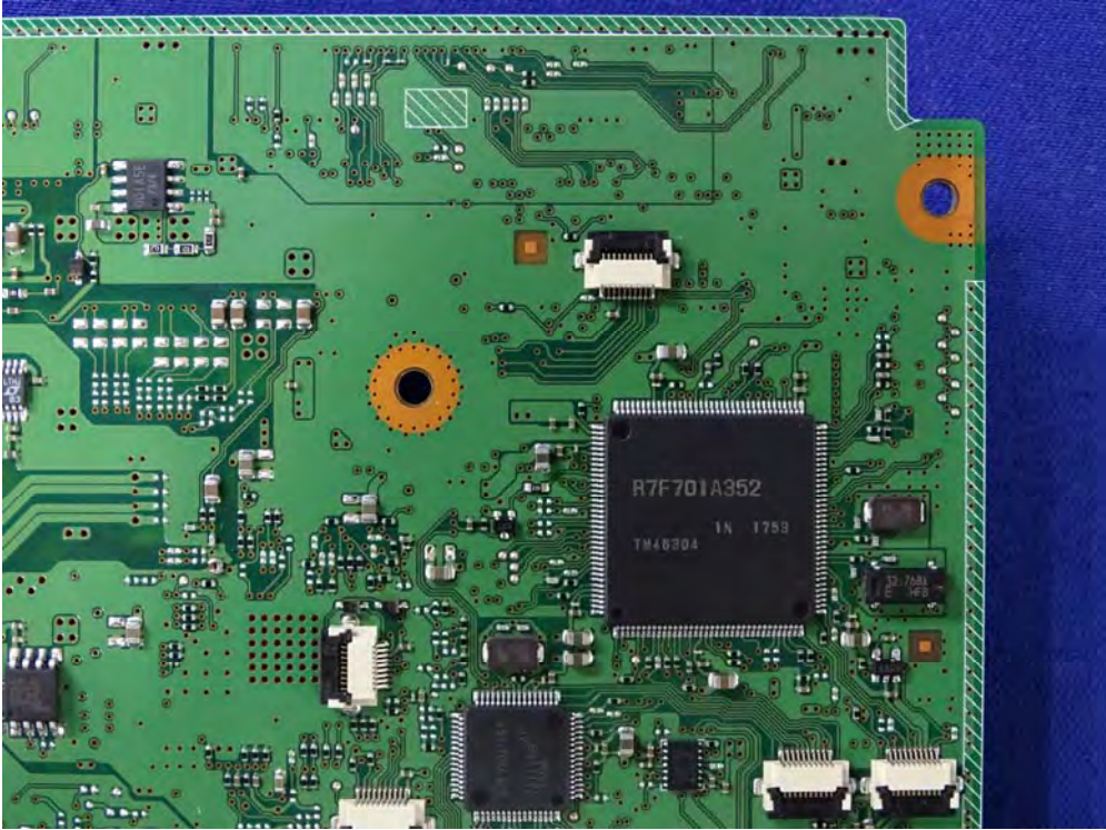
(74) EUT Photo
