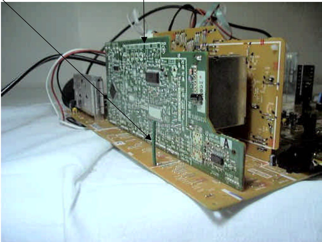
Lod Antenna
