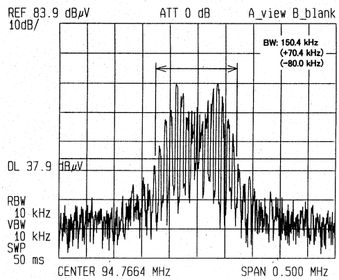
Audio input 1 kHz +8 dBV
